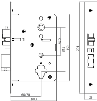
204*29mm ANSI mortise
