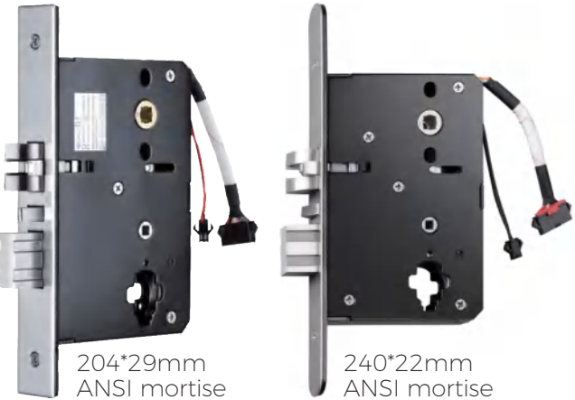
204*29mm ANSI mortise
