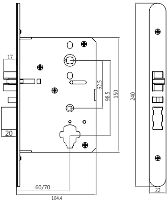
240*22mm ANSI mortise
