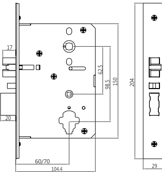
204*29mm ANSI mortise
