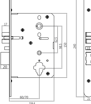
240*22mm ANSI mortise
